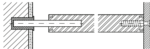
Verbindung Wand-Stufe
