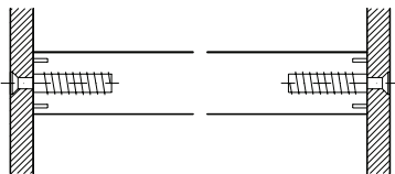
Verbindung Wange-Stufe
