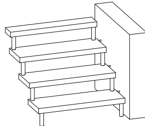
WF2 (1 Wandanker)
